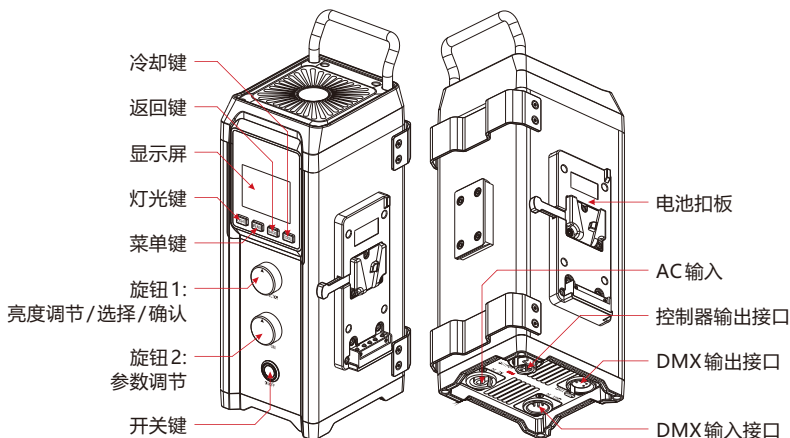
控制器
