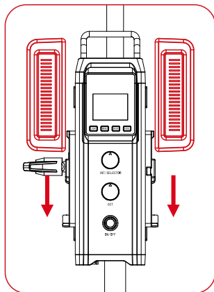
电池安装槽
